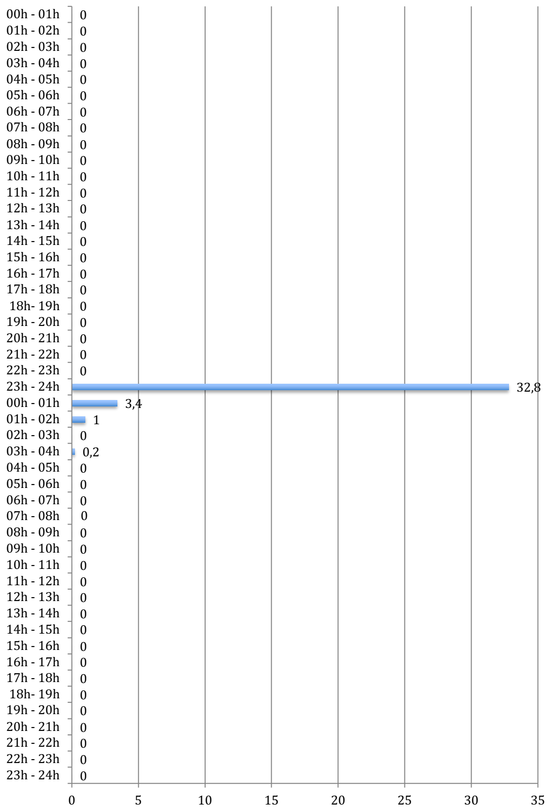
Cantidades de lluvia registradas por horas en SEDAVÍ el día 01 y 02/09/21 (en l/m²)
